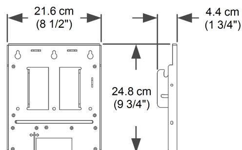
Support de fixation vue avant
