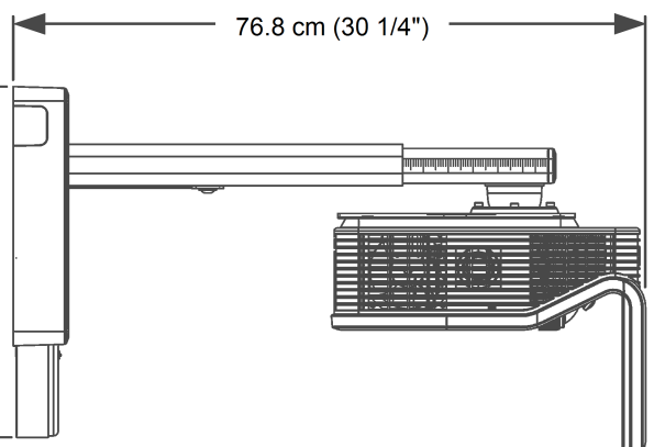
Vue latérale du projecteur interactif
