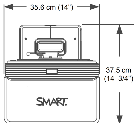
Vue avant du projecteur interactif
